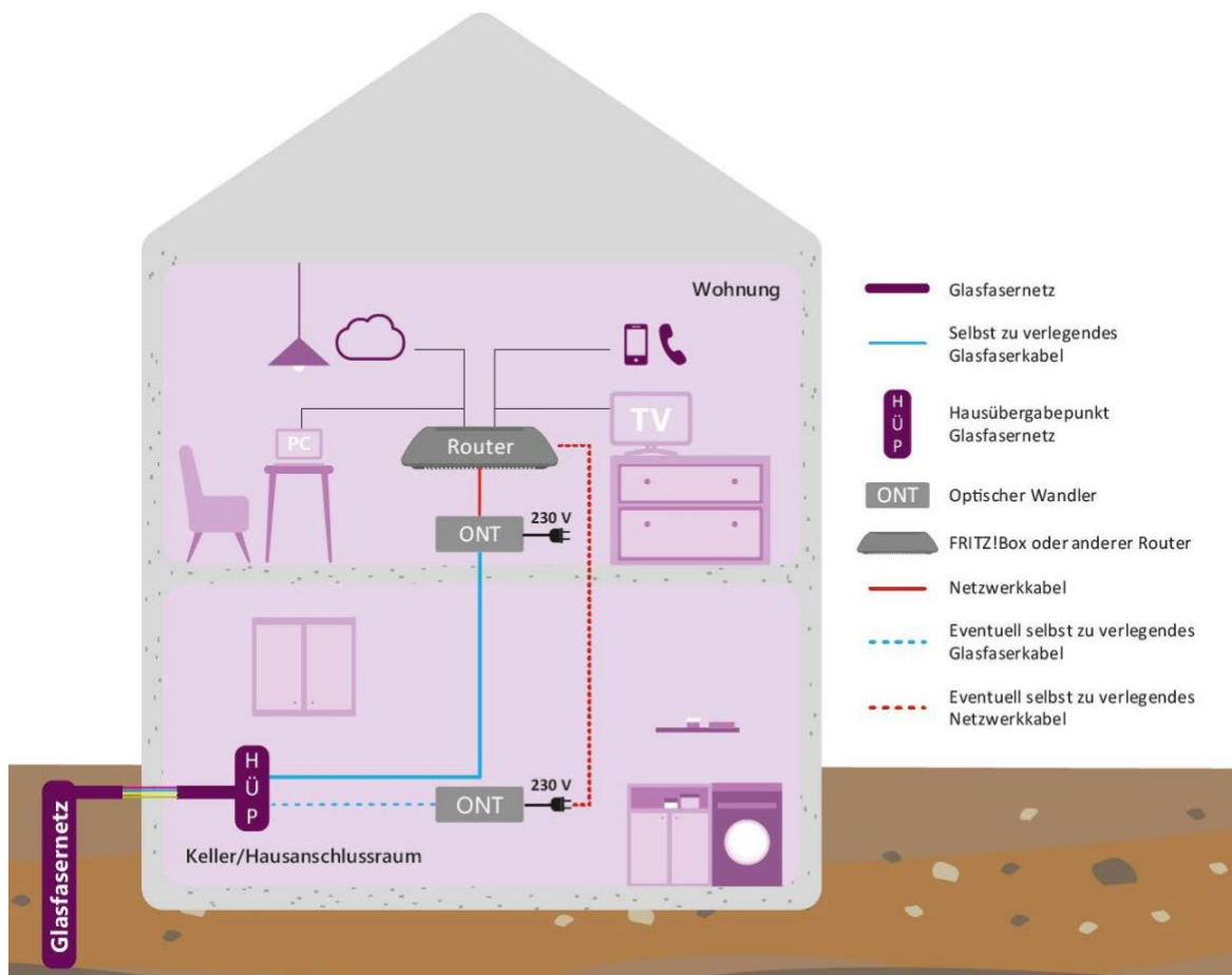
Abb. 1 Schema Verkabelung Ein- und Zweifamilienhaus
